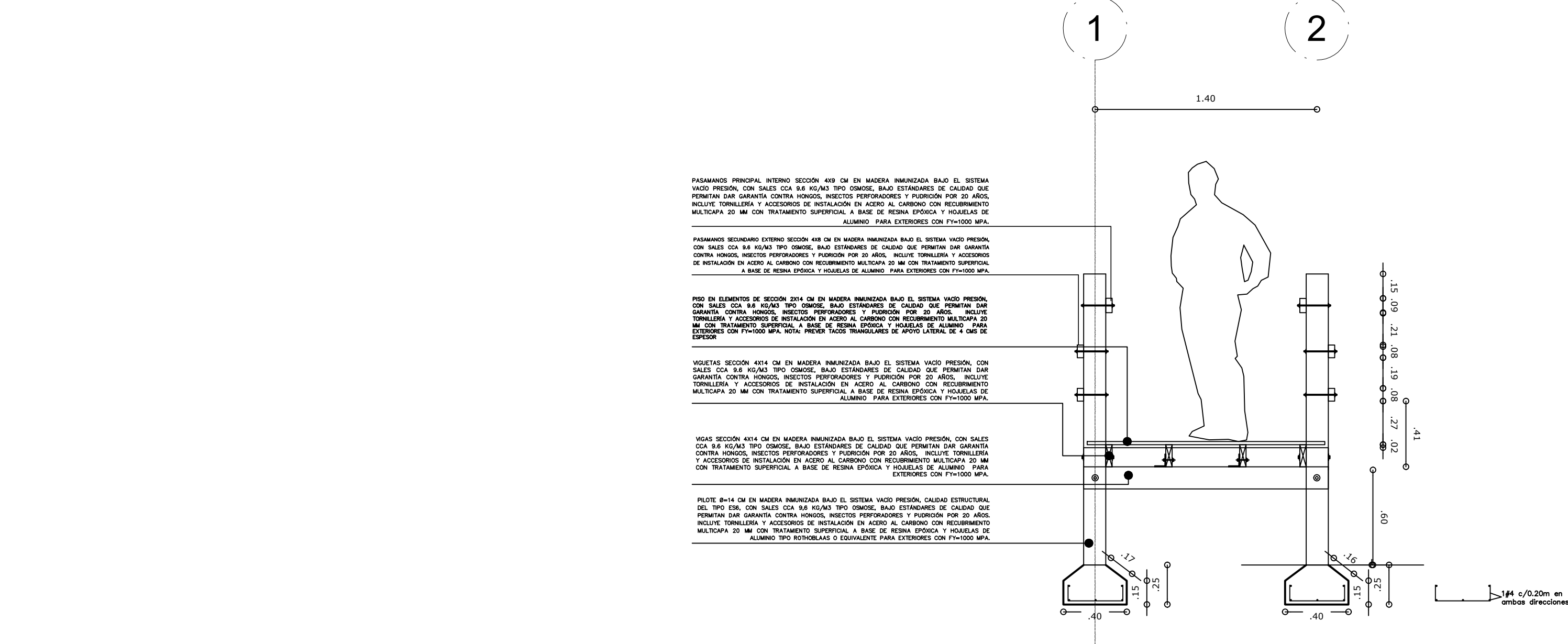
ESC - 1/25 CORTE TRANSVERSAL
