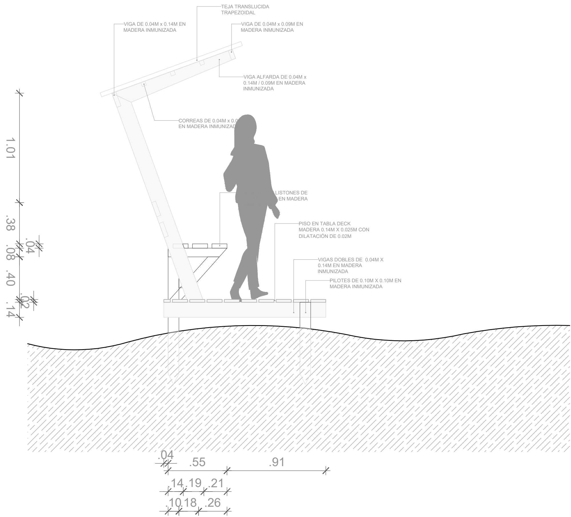
ZONA DE ESTANCIA CORTE B-B' - Esc 1:20
