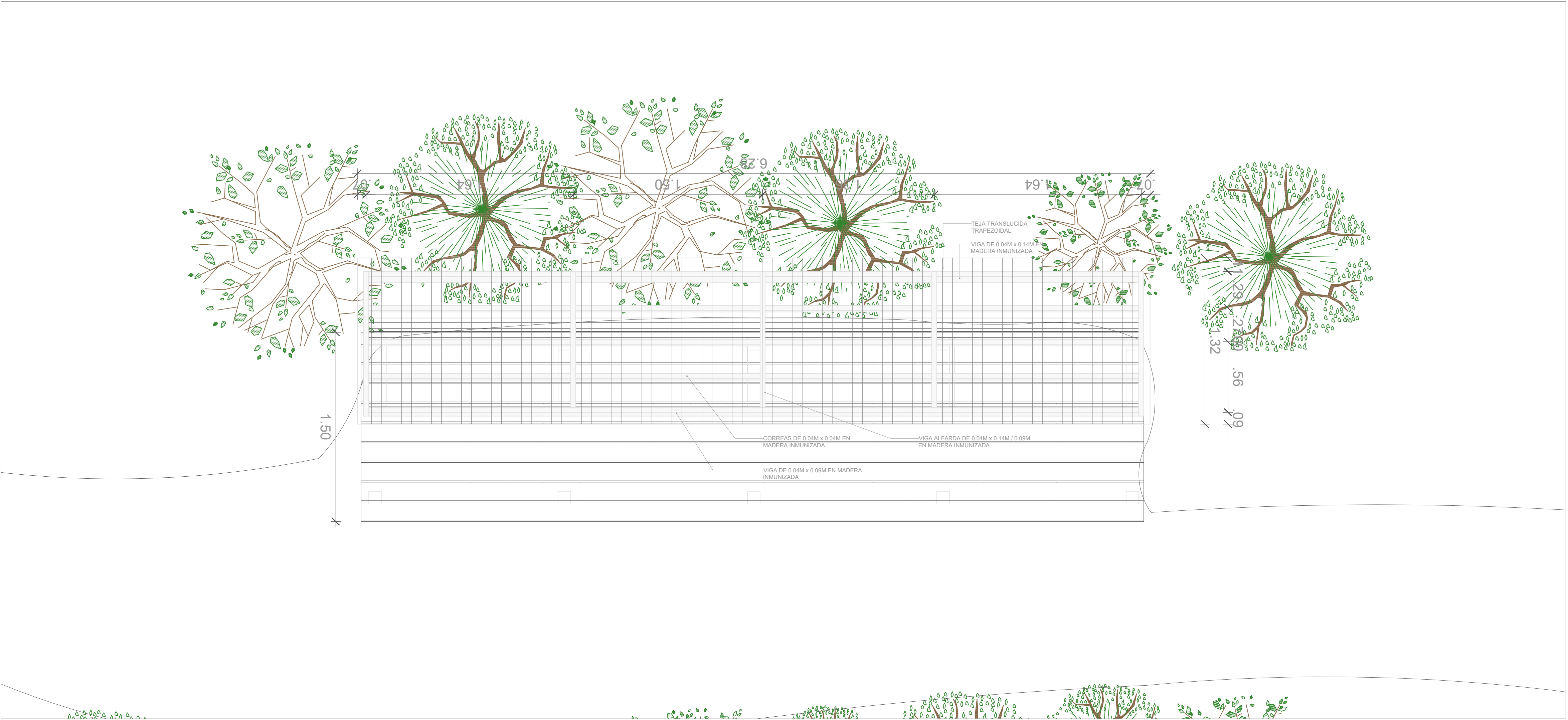
ZONA DE ESTANCIA PLANTA DE CUBIERTA - Esc 1:20
