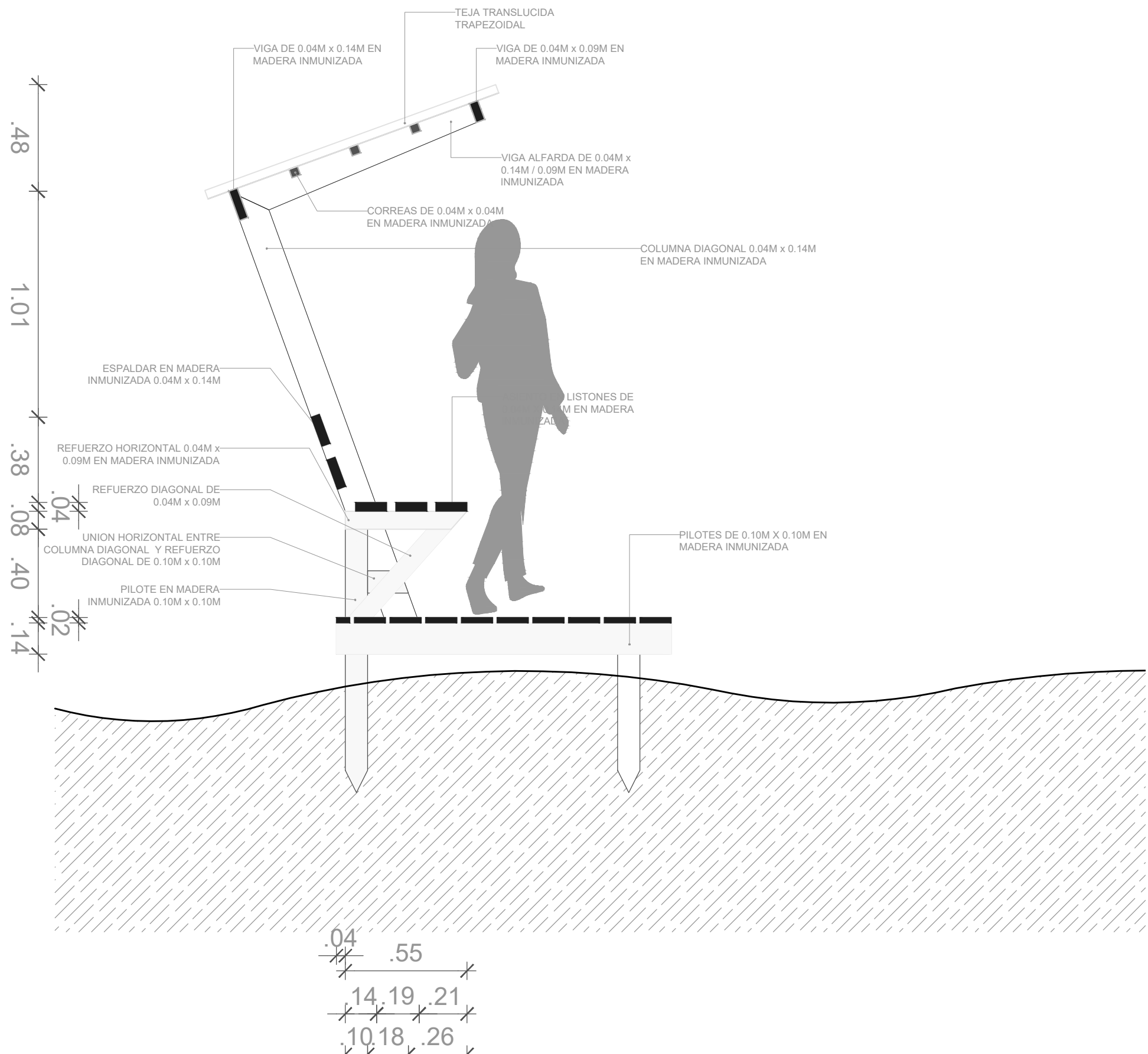
ZONA DE ESTANCIA CORTE A-A' - Esc 1:20
