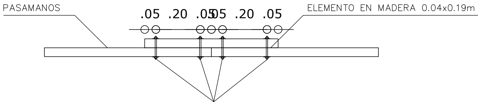
PLANTA DETALLE PARA UNIÓN DE PIEZAS QUE SUPERAN LOS 3m. 4+4 PERNOS Ø 1/2 CALIDAD B7 EN ACERO INOXIDABLE O GALVANIZADO
