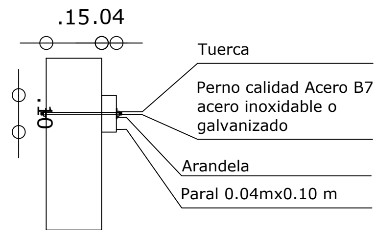
DETALLE PASAMANOS Y/ O DIAGONAL ESC: 1:10
