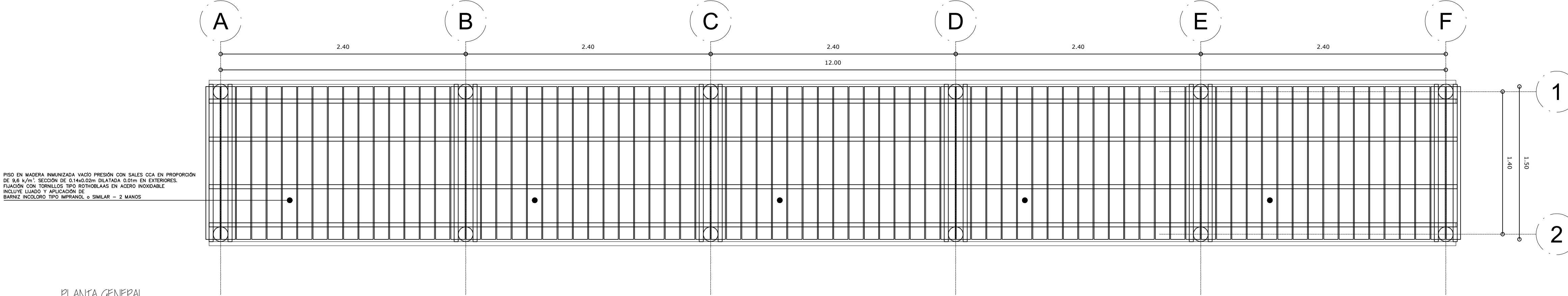
PLANTA GENERAL ESC - 1/25
