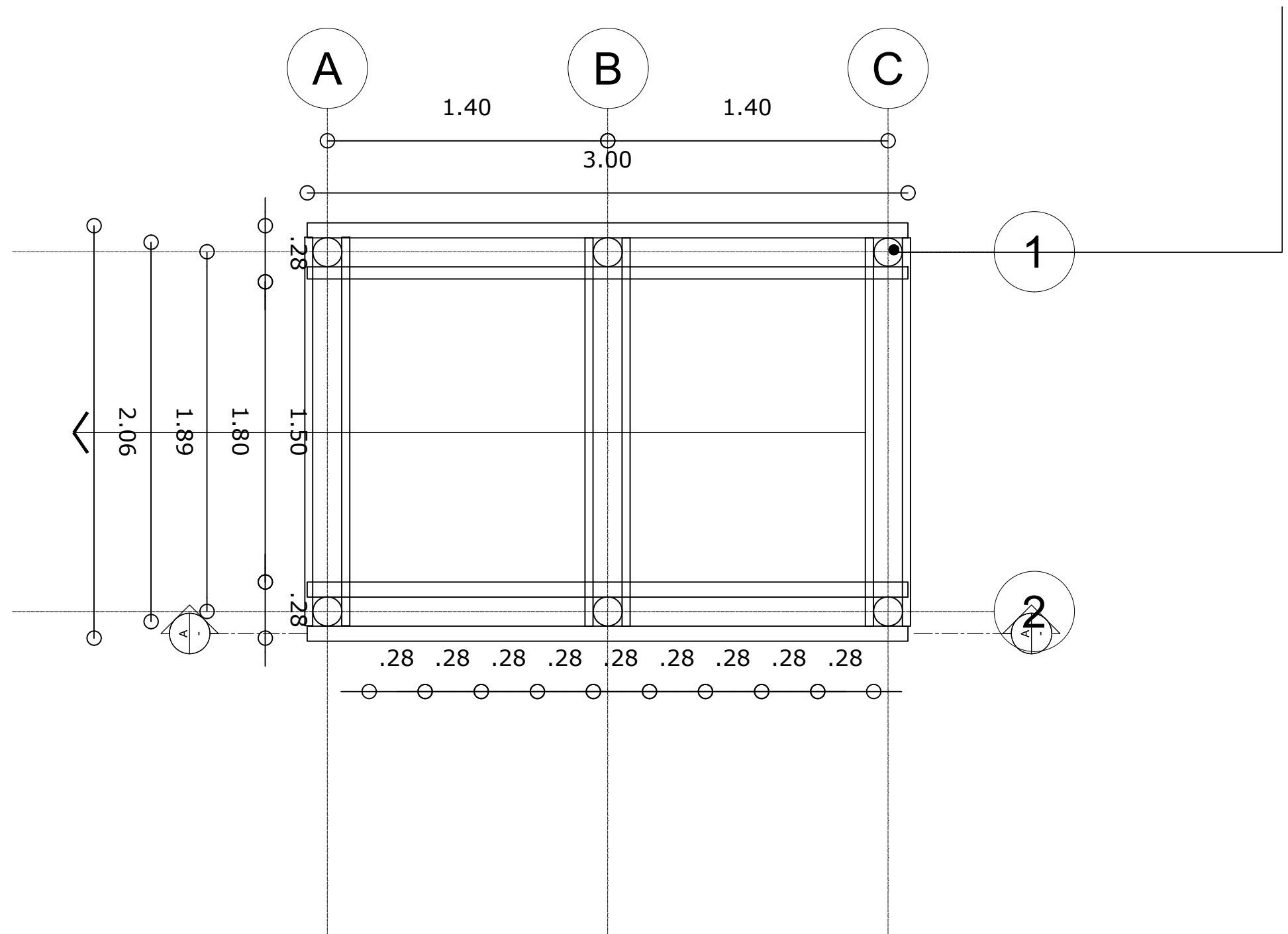
PLANTA ESTRUCTURA ESC - 1/25
