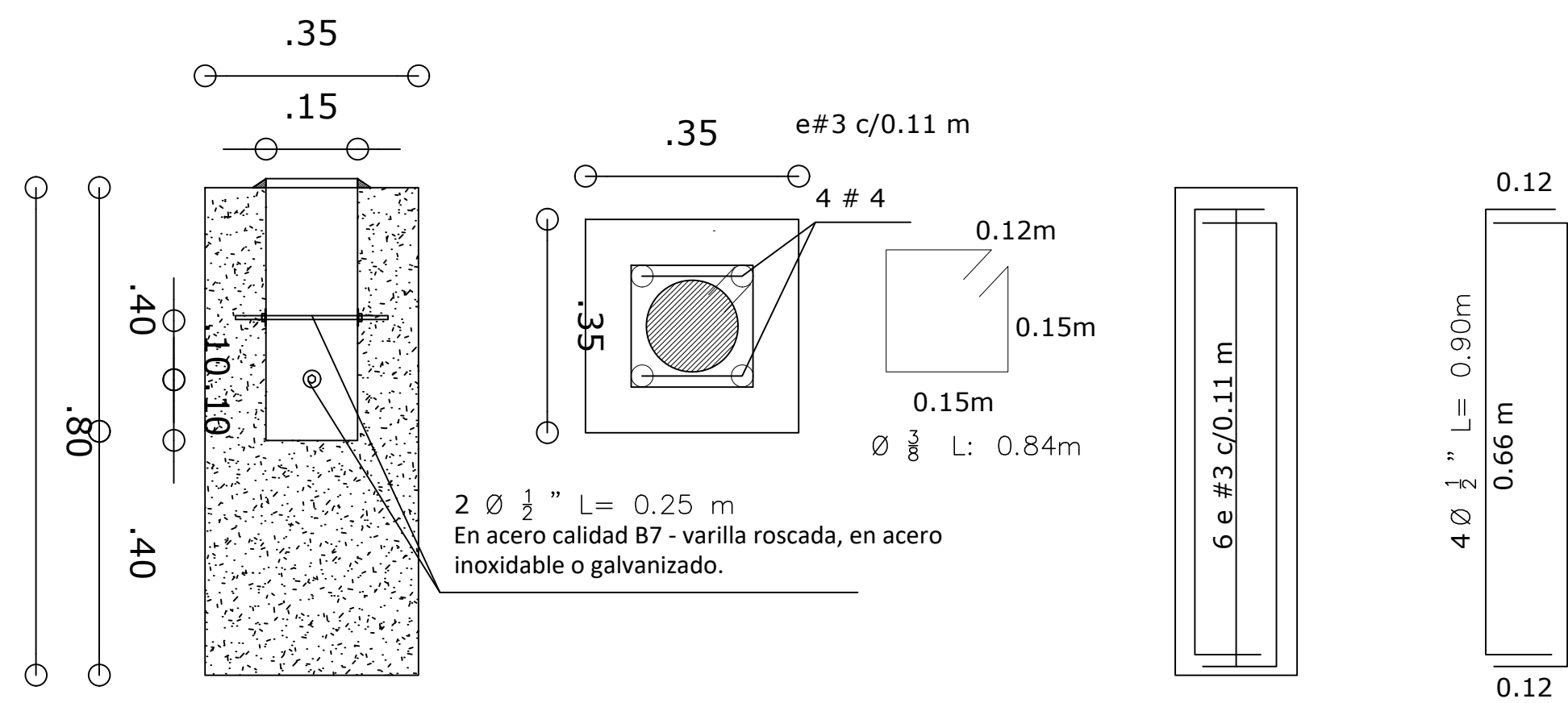
Detalle cimentación escalinata
