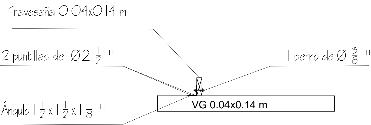
Detalle anclaje viguetas soporte ESC - 1/15 de listones
