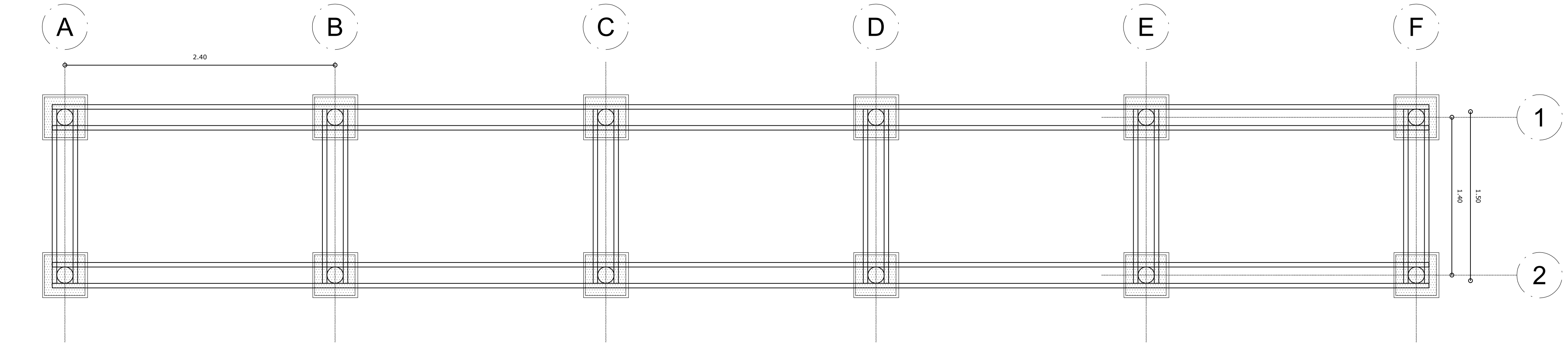
PLANTA CIMENTACIÓN
